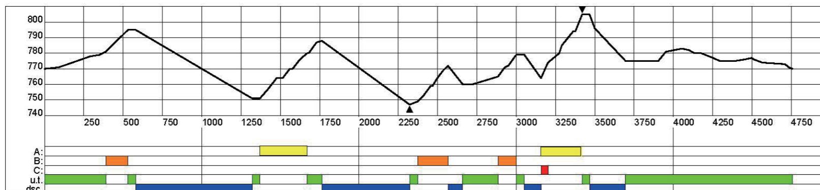
縦断面図
